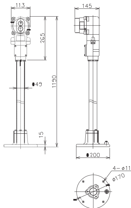
尺 寸 圖 單位 m
