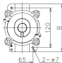
尺寸圖 單位 m
